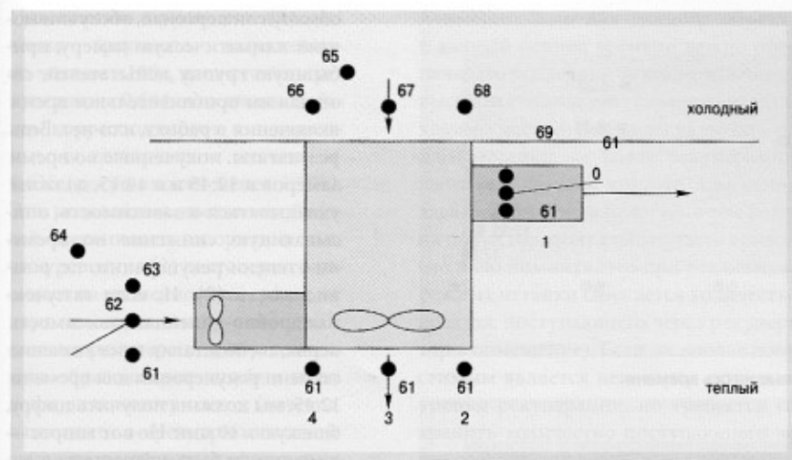
Рис. 1. Схема связей в единой технологической системе здания
