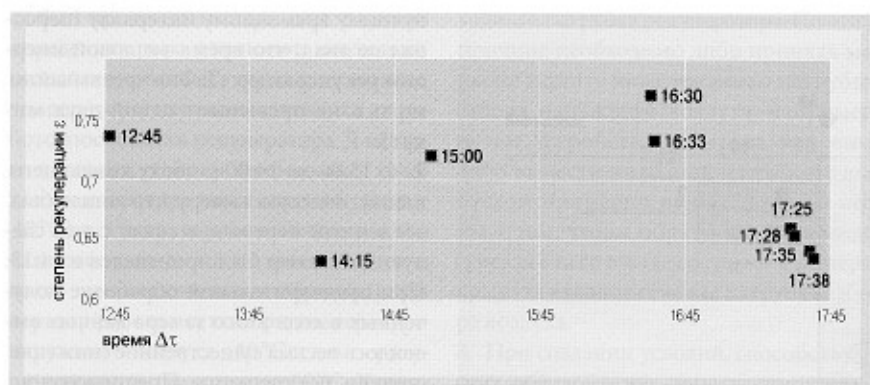
■ Рис. 2. Значения степени рециркуляции, положенные на ось времени
