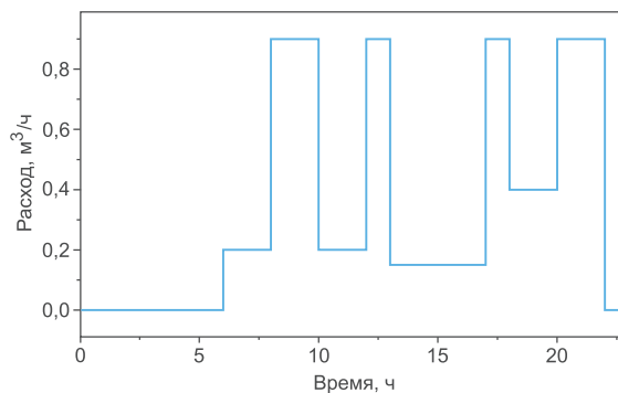
Рис. 1. График водоразбора на объектах с явно выраженной неравномерностью водопотребления.
