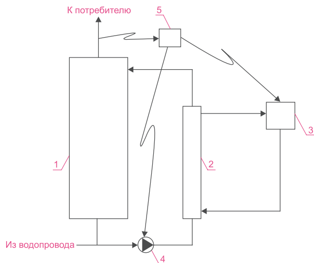
Рис. 2. Структурная схема емкостного водонагревателя с выносным греющим элементом:
